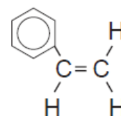
Styrene monomer
